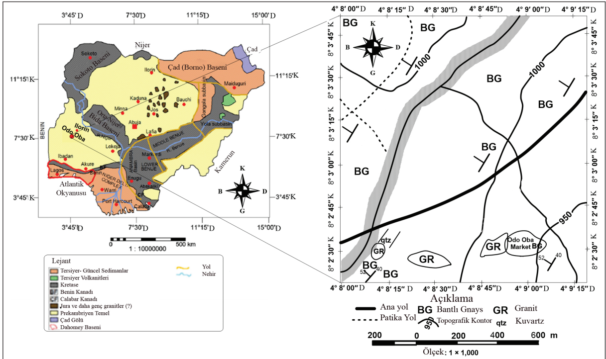
Şekil 2- Nijerya'daki jeolojik birlikeliler ve Odo-Oba bölgesinin jeoloji haritaları (Obaje, 2015; Adagunodo vd., 2017b, 2018c).
