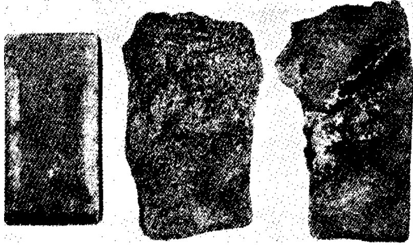
No. 1 Siemens-Martin çelik fırınlarında fazla kullanılan krom-magnesium tuğla sathının tedricen süngerleşmesi. Yeni tuğla Müstamel tuğla
